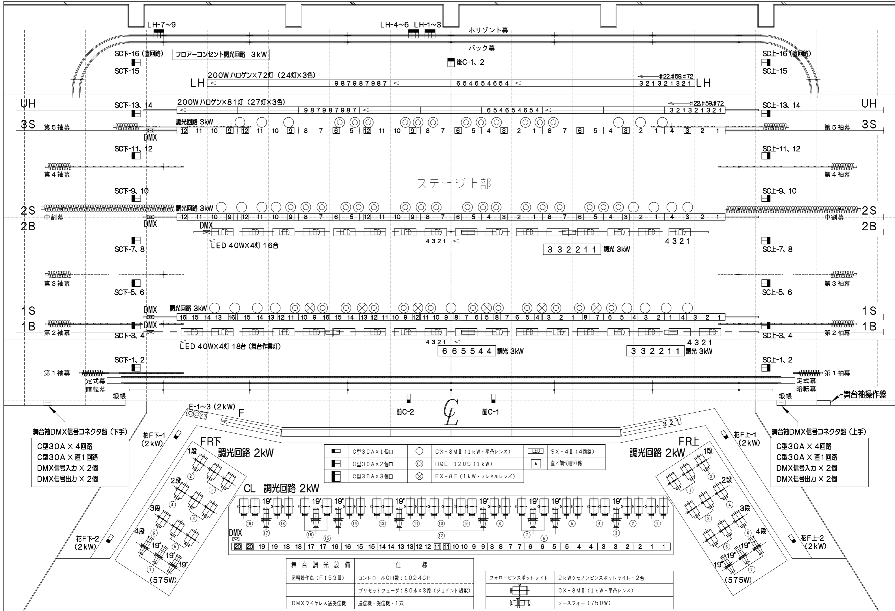
【利根沼田文化会館 大ホール 照明配置図】
